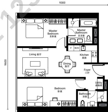
D-1 2 BEDROOMS 卧室 84 SQ.M. 903 SQ.FT. 平方米 平方尺
