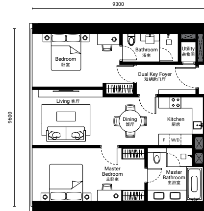
D-3 DUAL KEY 双钥匙 89 SQ.M. 956 SQ.FT. 平方米 平方尺
